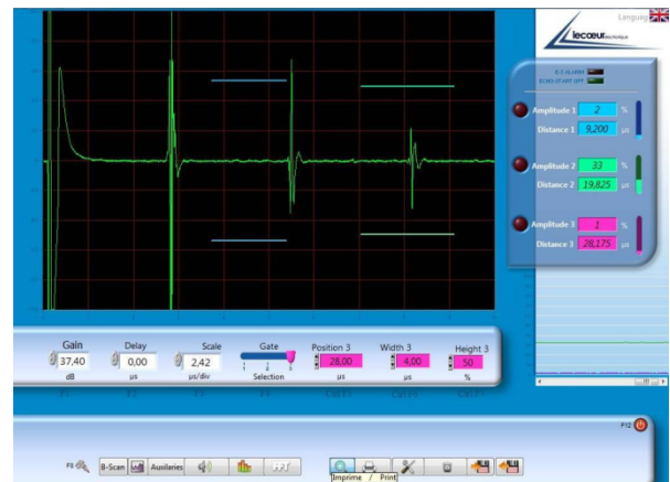
RF表示、VIDEO表示ほか、DAC,Bスコップ表示等探傷器機能を満載
