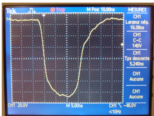
スクエアタイプパルサー 20~230V(50Ω負荷)
