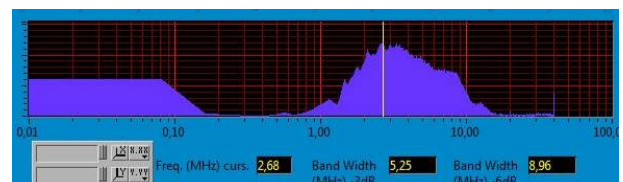
FFT解析画面
